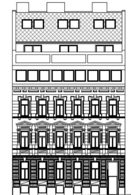
STRASSENFASSADE M1:200
