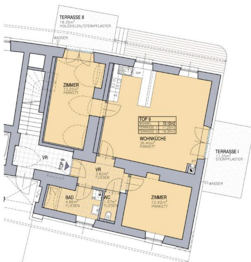
GRUNDRISS ERDGESCHOSS
