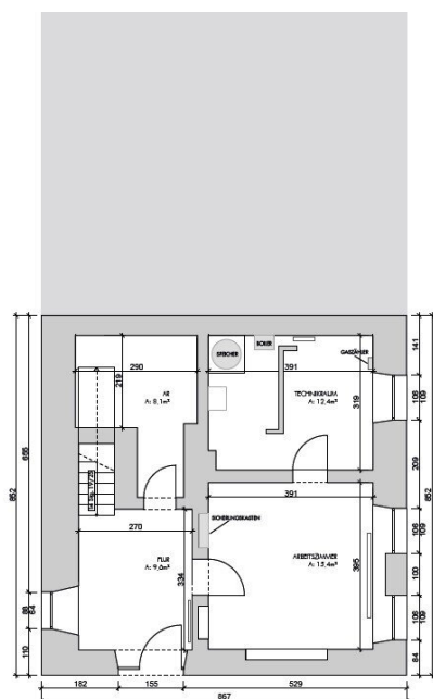
GRUNDRISS EG M1:100
