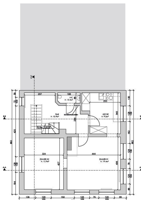
GRUNDRISS OG1 M1:100
