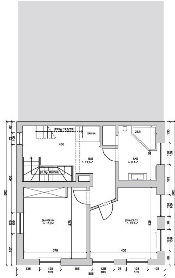
GRUNDRISS OG2 M1:100
