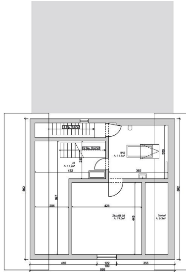
GRUNDRISS DG M1:100
