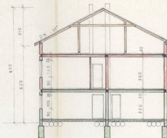
SCHNITT A-A
