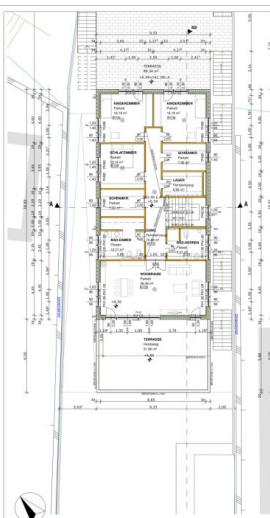
GRUNDRISS 1. OBERGESCHOSS M 1:100
