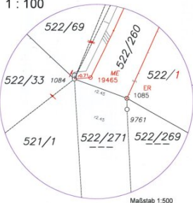
Detail 1 1 : 100
