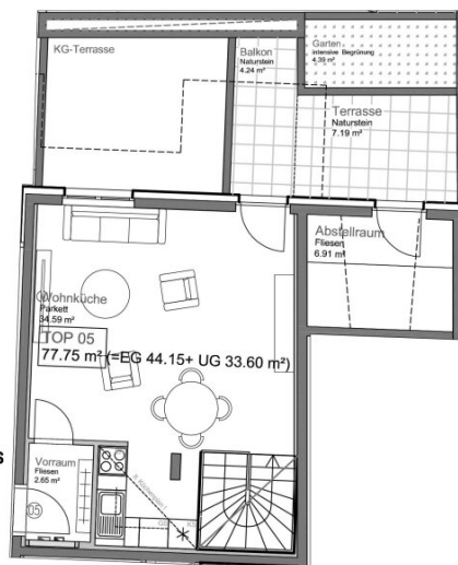
ERDGESCHOSS ST-TOP 05
