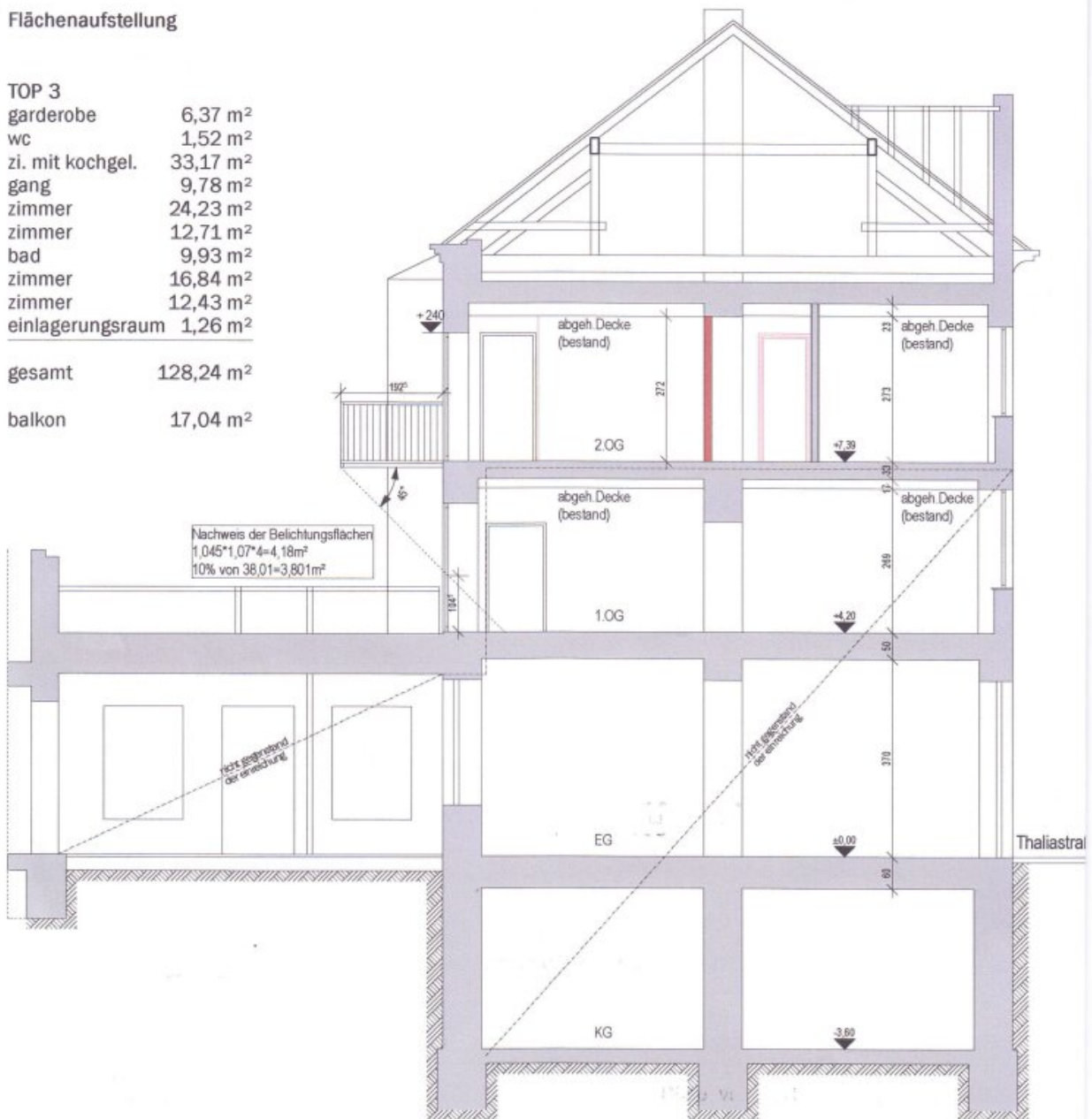
Schnitt a-a
