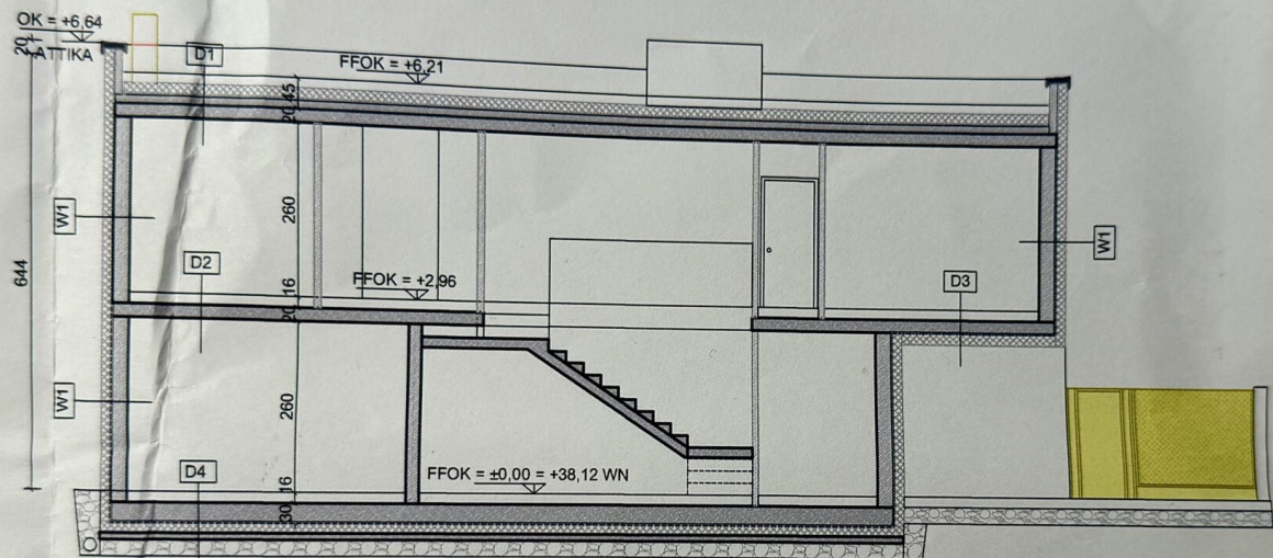
SCHNITT "A"
