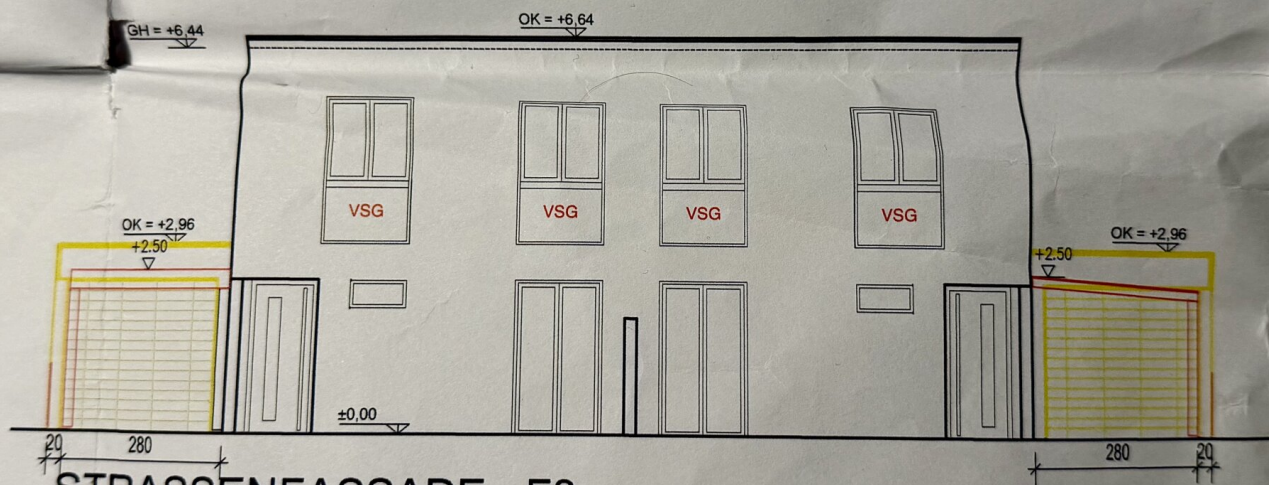
STRASSENFASSADE - F3
