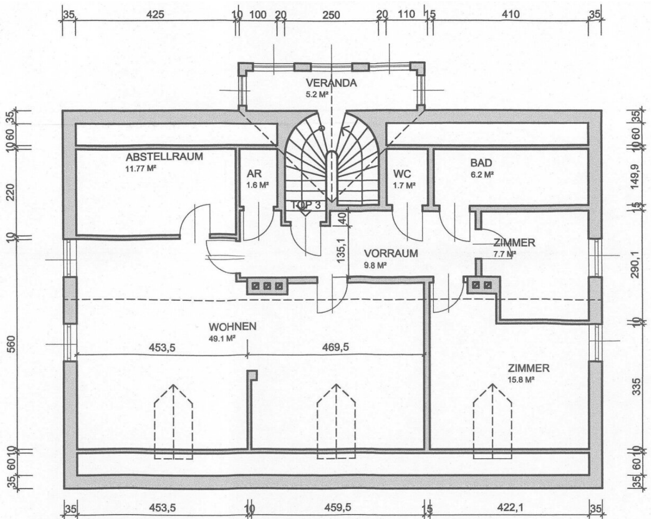
DACHGESCHOSS M 1:100
