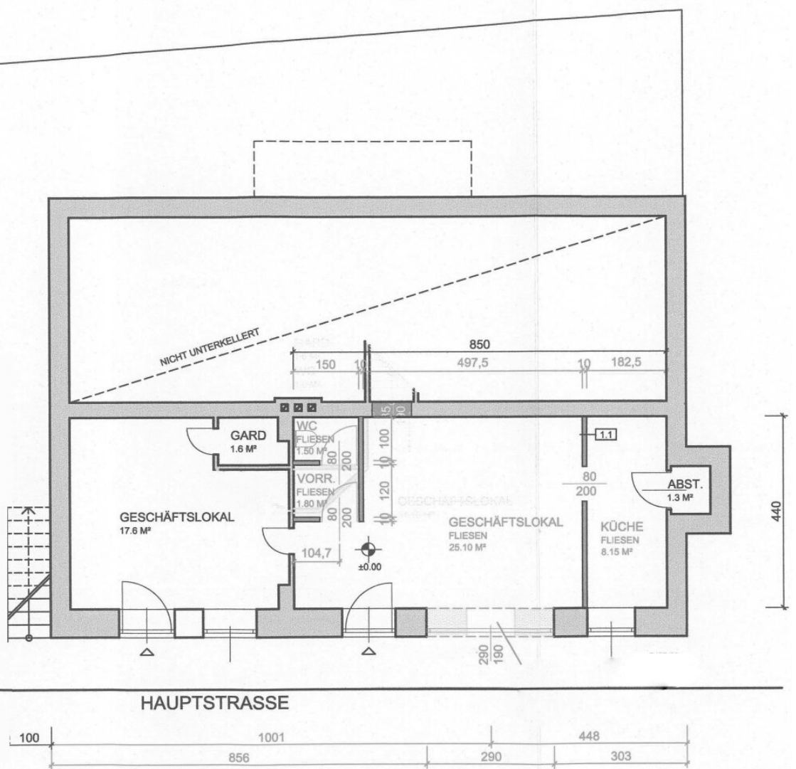
ERDGESCHOSS M 1:100
