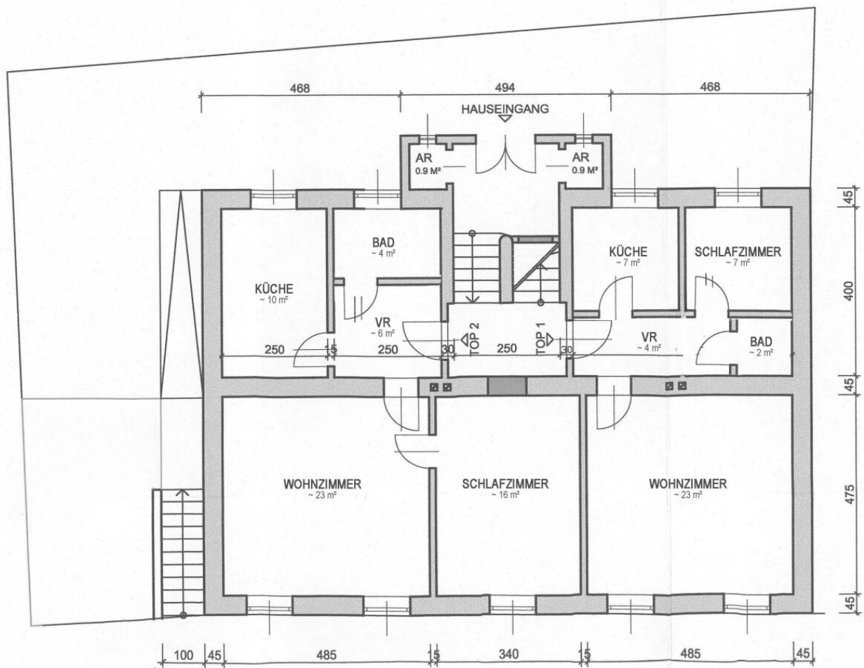
OBERGESCHOSS M 1:100
