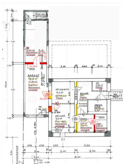
KELLERGESSCHOSS
