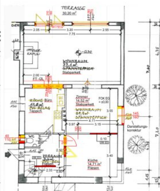
ERDGESCHOSS
