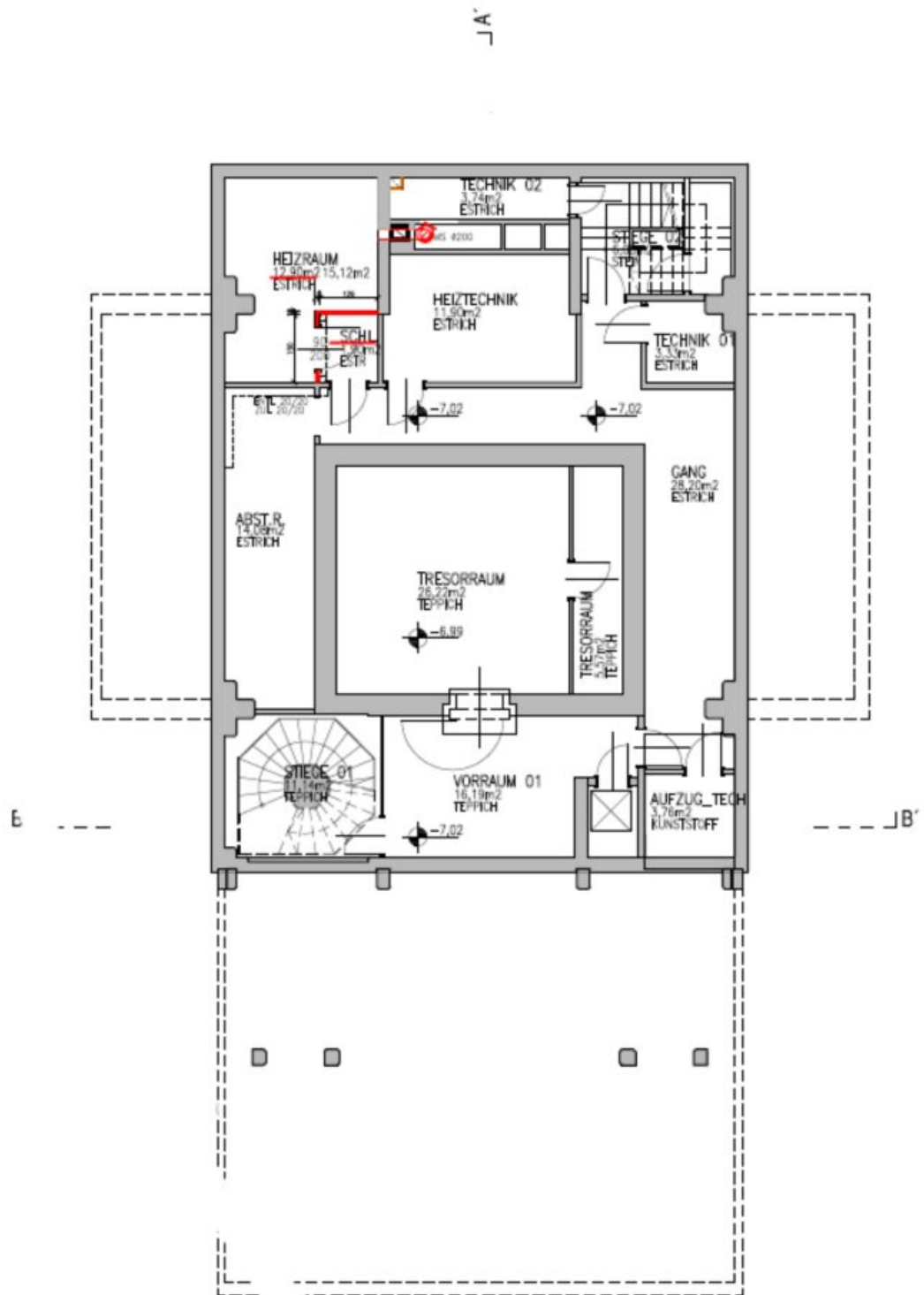
GRUNDRISS 2.KELLERGESCHOSS
