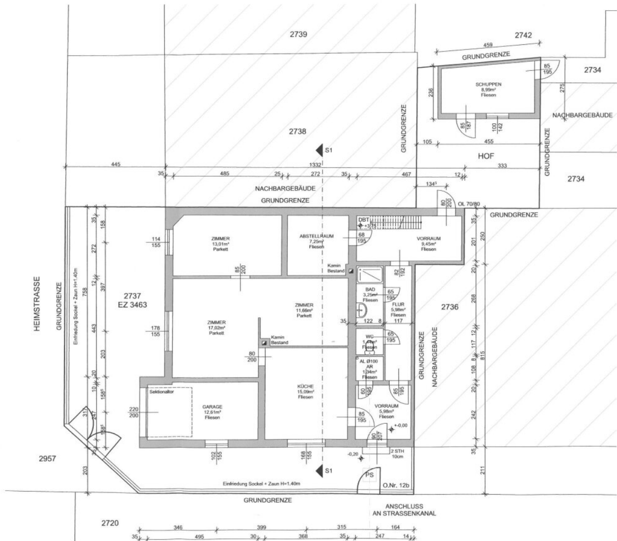
GRUNDRISS ERDGESCHOSS
