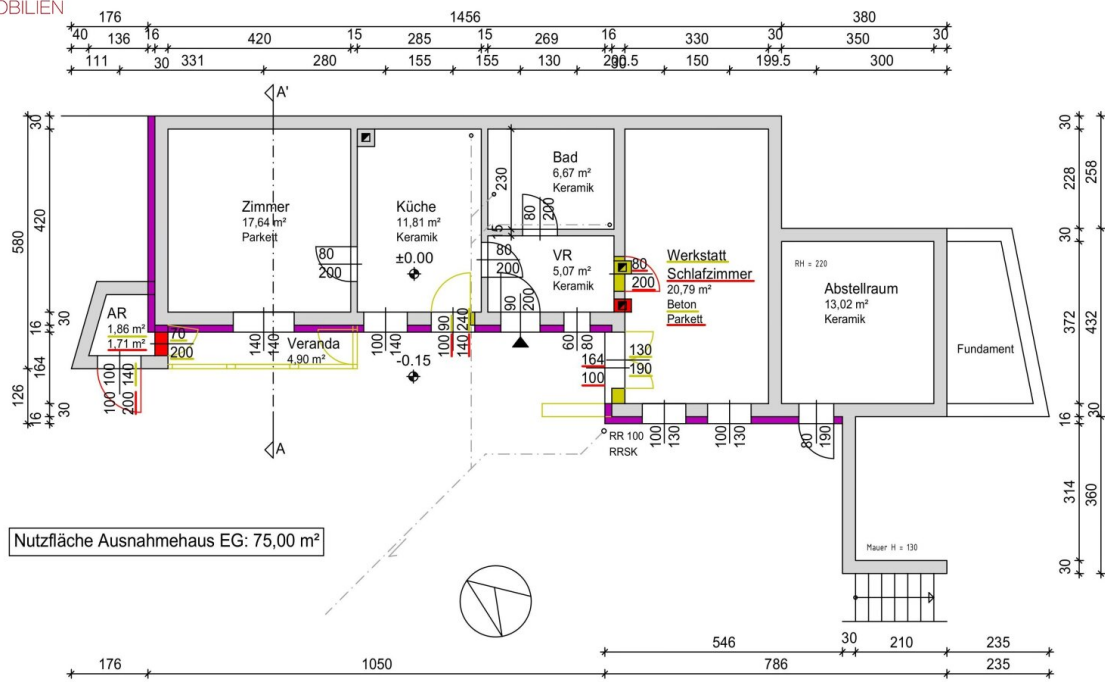
AUSNAHMEHAUS GRUNDRISS EG M=1:100
