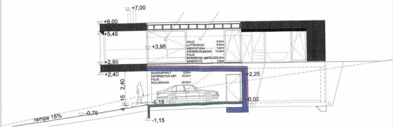
schnitt b
