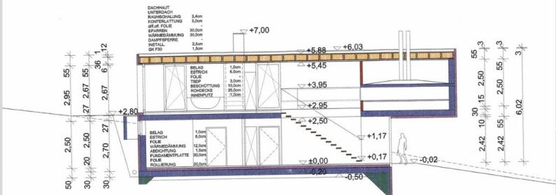
schnitt b
