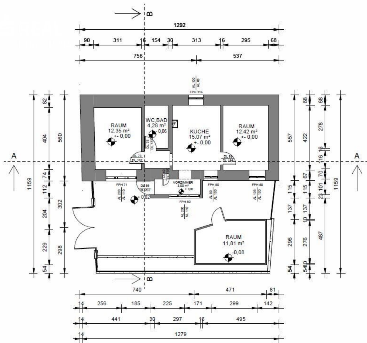
GRUNDRISS ERDGESCHOSS
