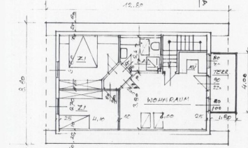
DACHGESCHOSSGRUNDRISS
