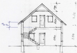
SCHNITT A-B
