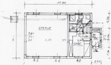
ERDGESCHOSSGRUNDRISS
