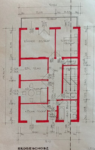
ERDGESCHOSZ
