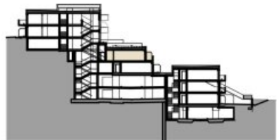
SCHNITT BK 02+04
