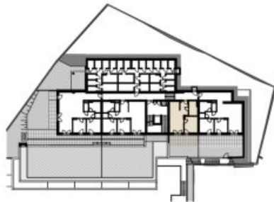
GRUNDRISS BK 04
