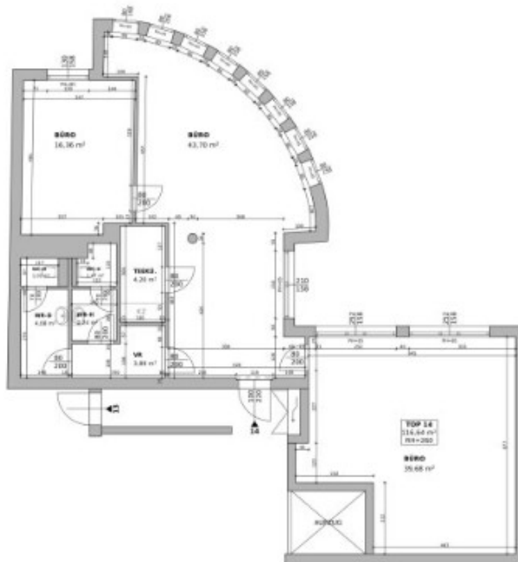
GRUNDRISS STIEGE 2 4. OBERGESCHOSS TOP 14
