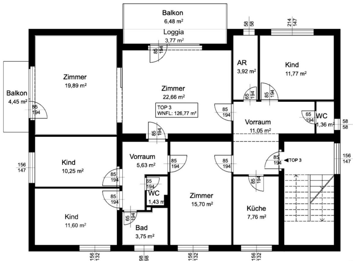
Grundriss Skizze
