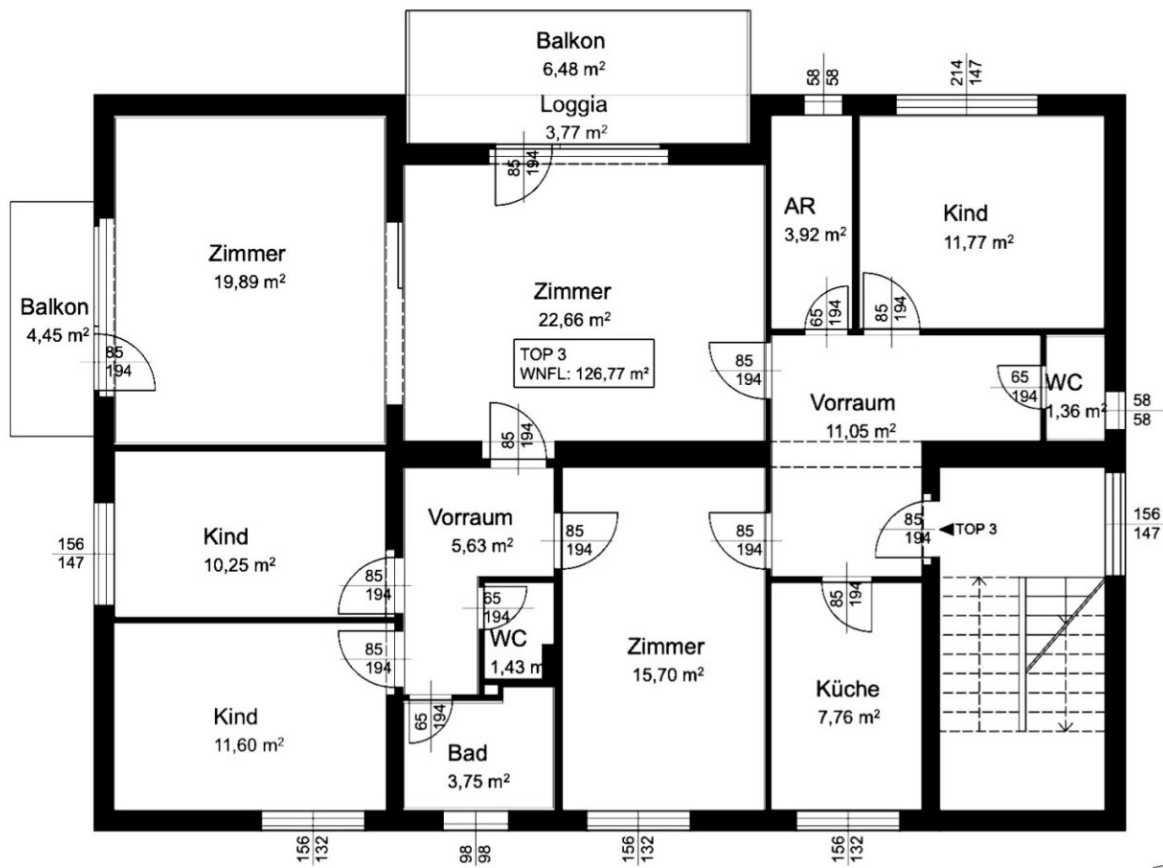
Grundriss Skizze
