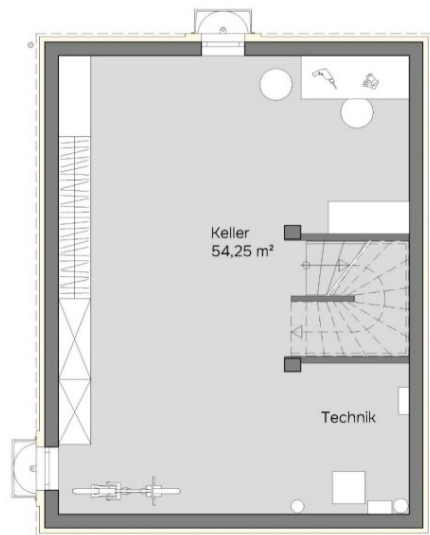
Kellergeschoss Raumhöhe 2.22 m
