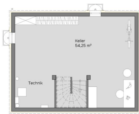
Kellergeschoss Raumhöhe ≈ 2,20 m
