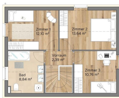
Obergeschoss
