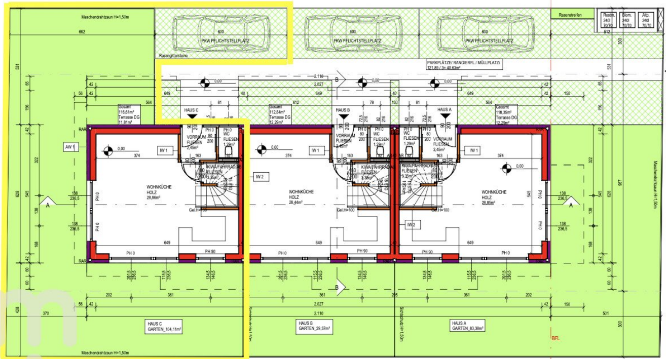
ERDGESCHOSS
