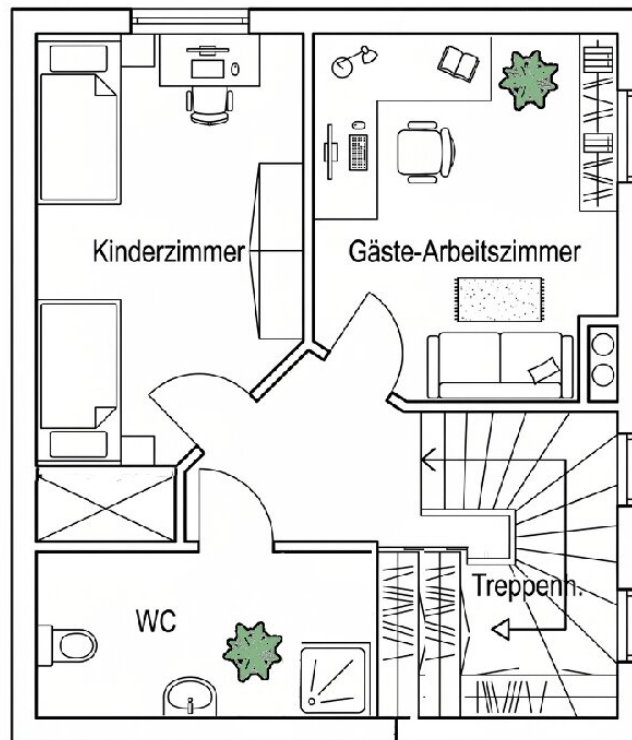
Obergeschoss
