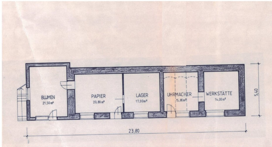
Grundriss Untergeschoss
