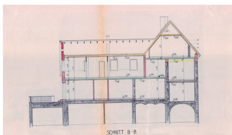
Schnitt
