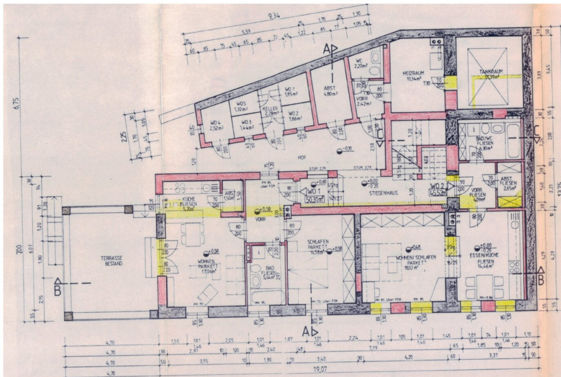
Grundriss Erdgeschoss 2 Wohneinheiten
