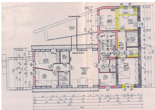
Grundriss Obergeschoss 2 Wohneinheiten
