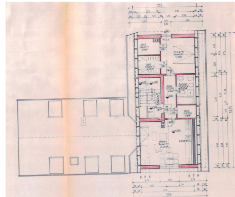
Grundriss Dachgeschoss 1 Einheit
