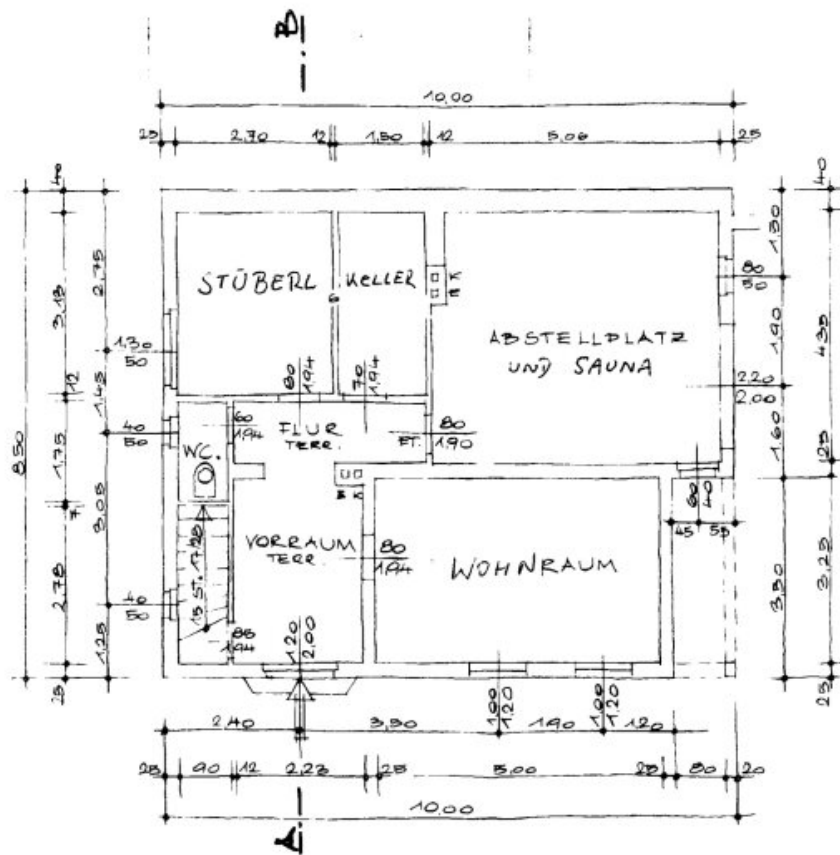
ERDGESCHOSS
