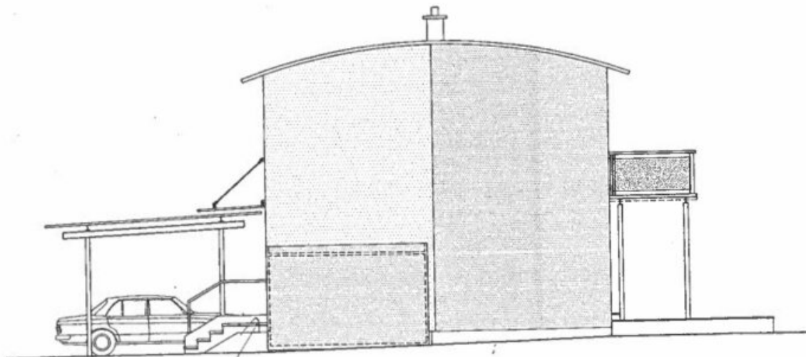
NORDWESTANSICHT
