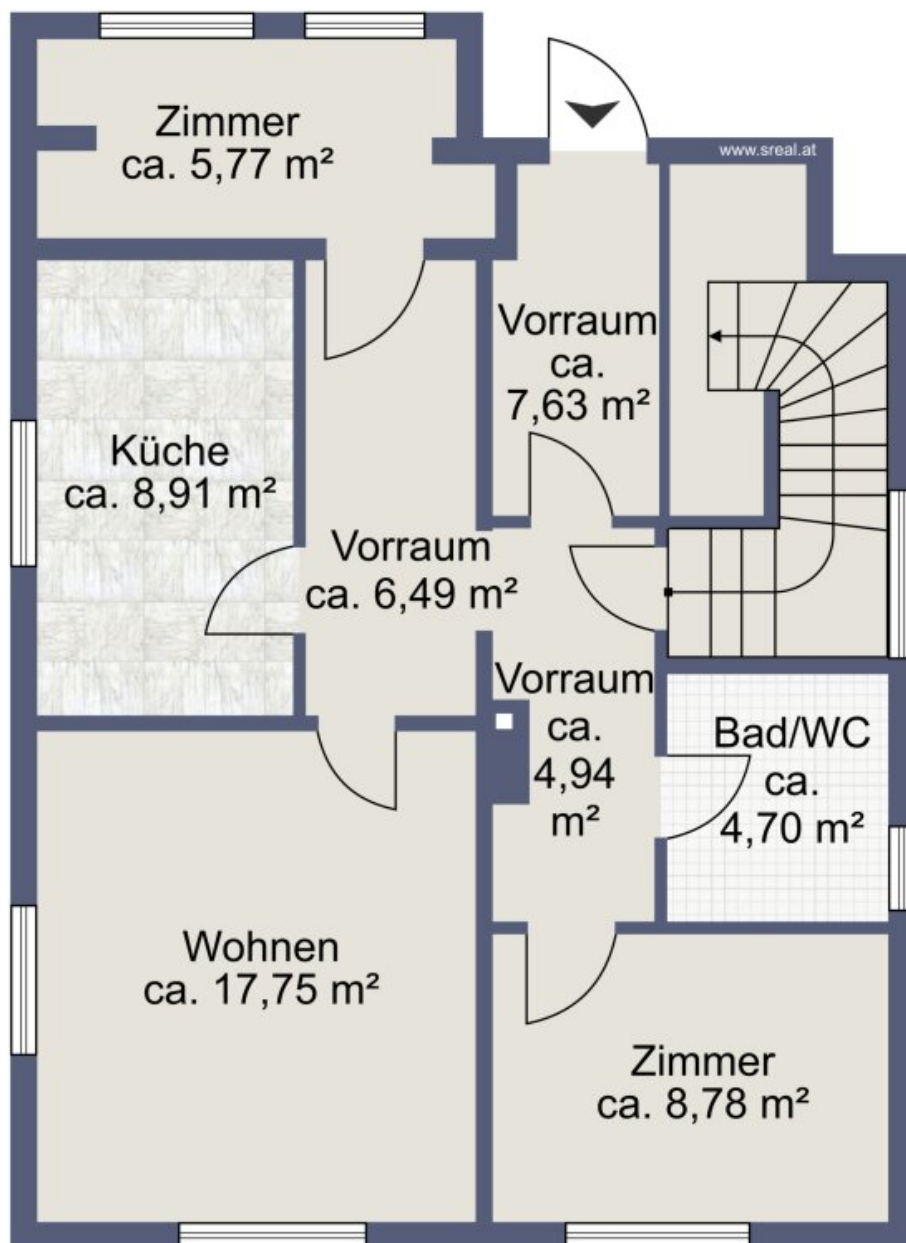
Skizze Erdgeschoss
