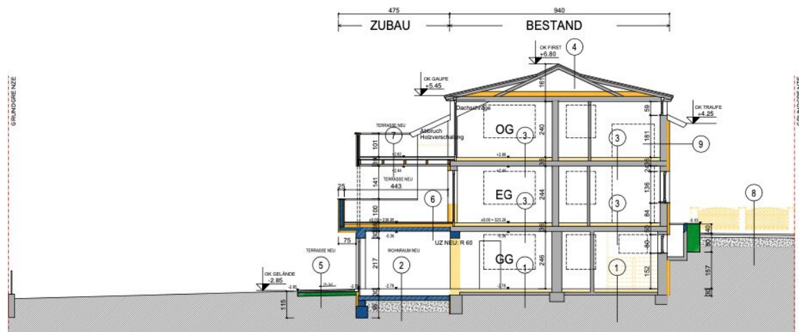
SNITT A-A
