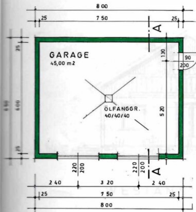
GRUNDRISS
