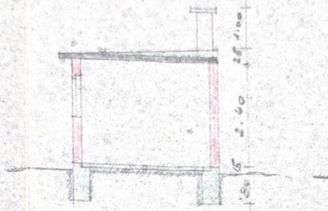
SCHNITT C:D
