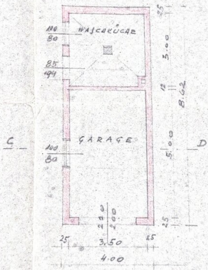
GRUNDRISS
