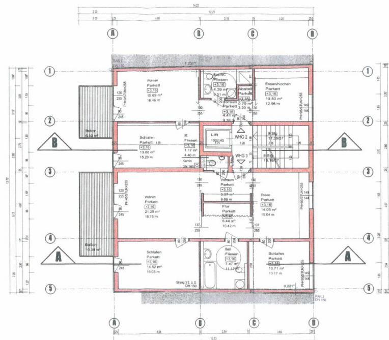
1.0BERGESCHOSS
