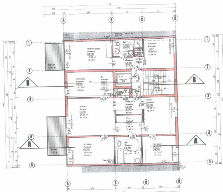
2.OBERGESCHOSS
