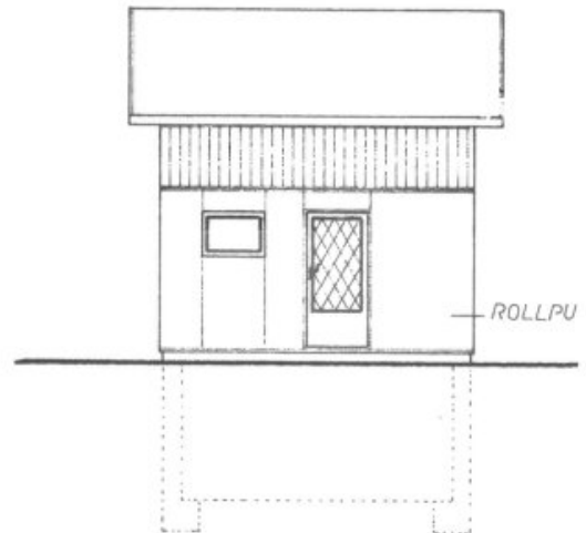
O ANSICHT
