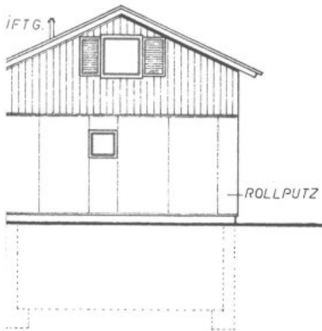
N ANSICHT
