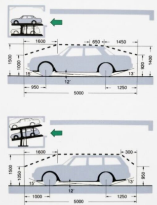
Zugelassene PKW-Maße für die Standardanlage
