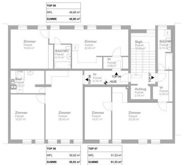
2. OBERGESCHOSS | 1:100
