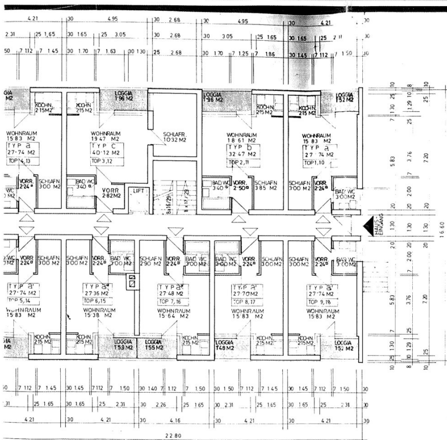
d-u. 1. obergeschoss
