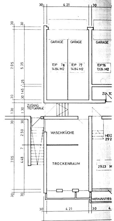
kellergeschoss
