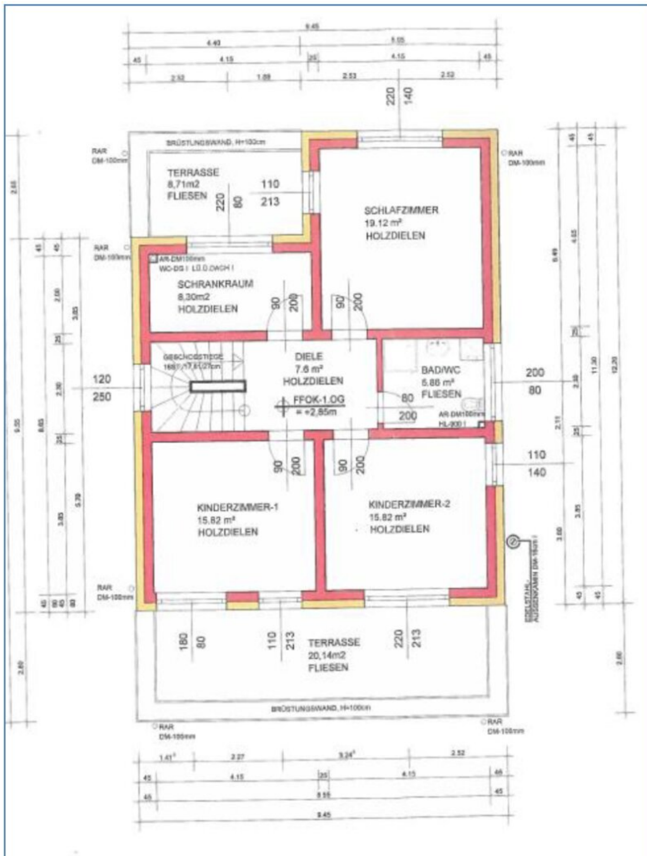
Grundriss 1. OG
