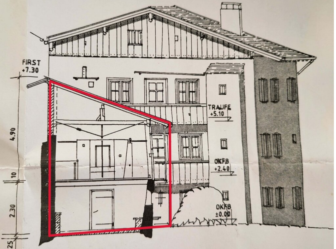
SCHNITT A-A
