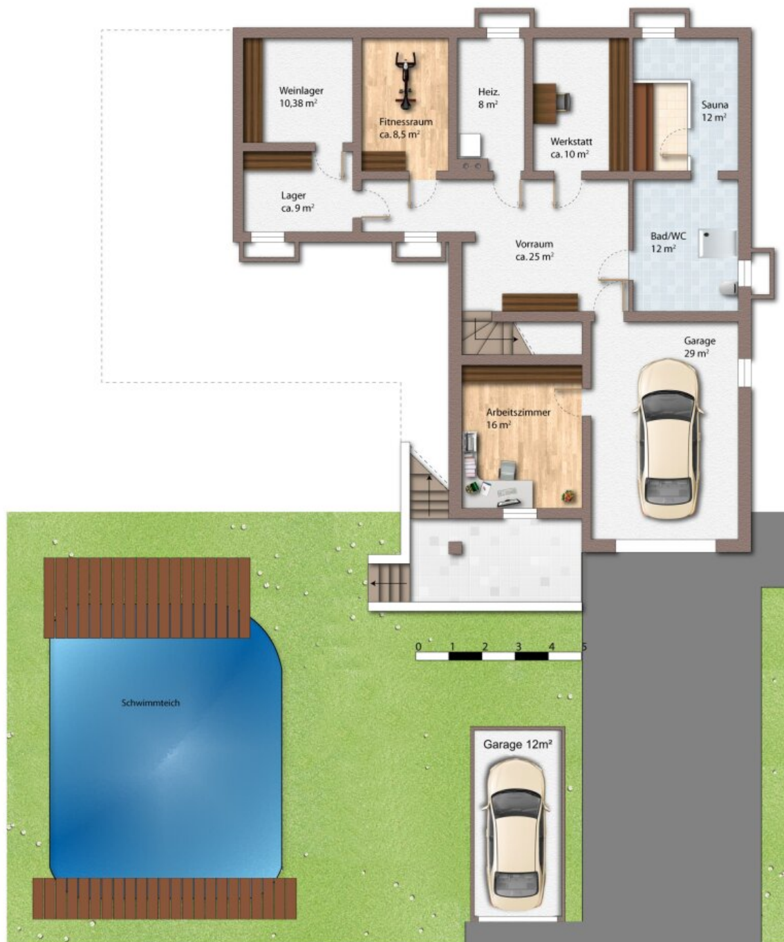
Grundriss Untergeschoss
