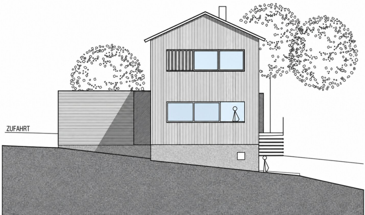
ANSICHT WESTEN M 1:100
