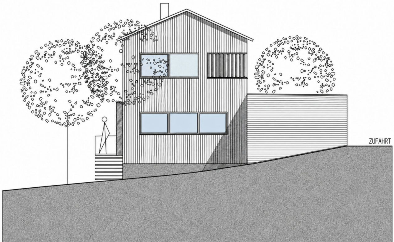
ANSICHT OSTEN M 1:100
