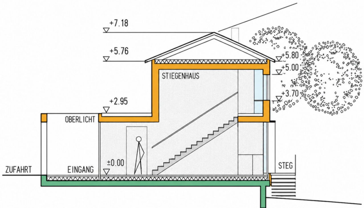
SCHNITT 1-1 M 1:100
