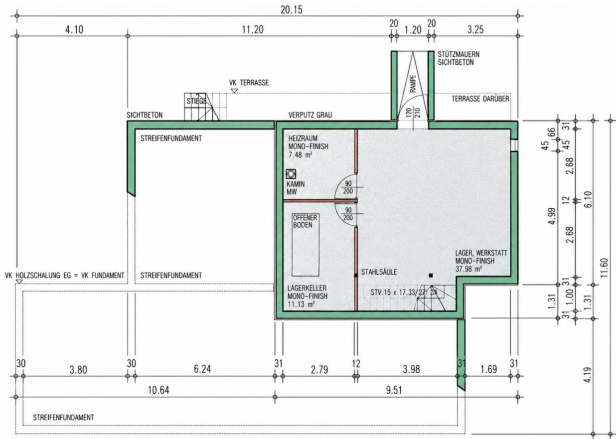
KELLERGESCHOSS M 1:100
