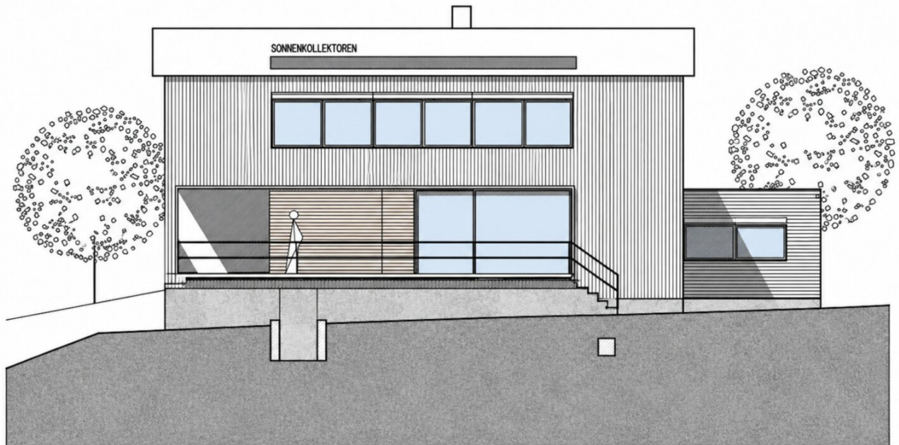
ANSICHT SÜDEN M 1:100
