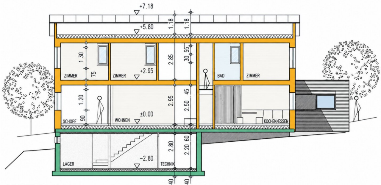
SCHNITT 2-2 M 1:100
