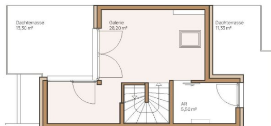
Dachgeschoss
