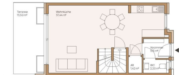
Erdgeschoss
