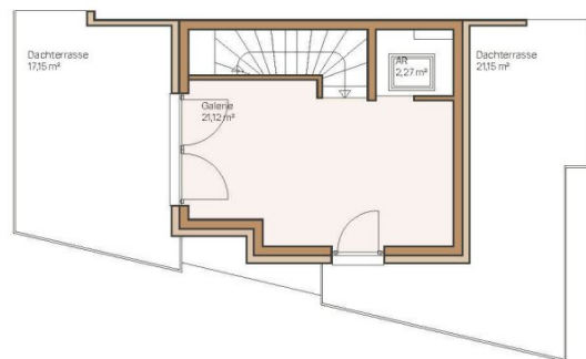
Dachgeschoss
