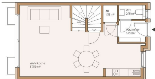
Zweites Geschoss
