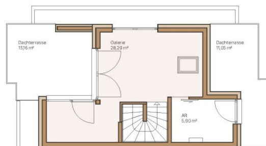
Dachgeschoss
