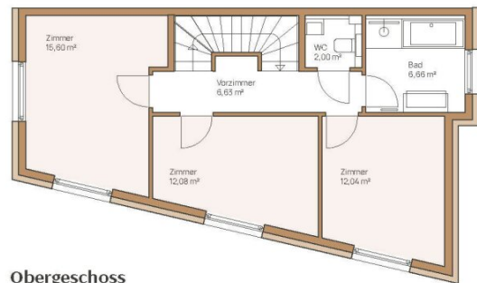
Obergeschoss
