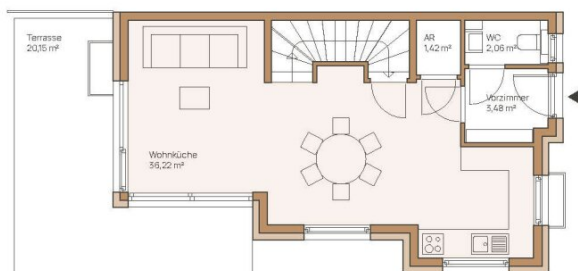
Erdgeschoss
