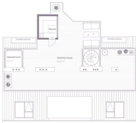
Dachdraufsicht
