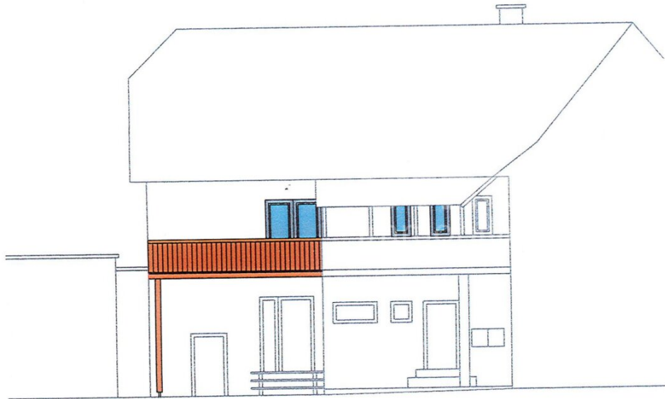
Ansicht Nord M: 1:100
