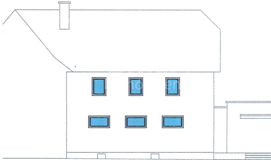
Ansicht Süd M: 1:100
