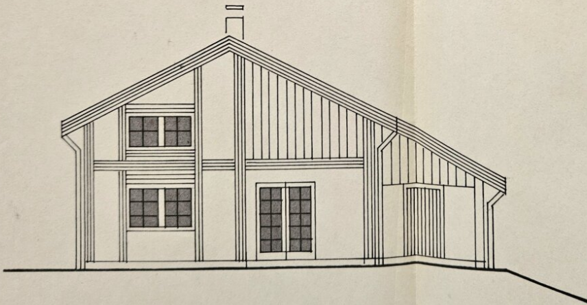
ANSICHT WEST
