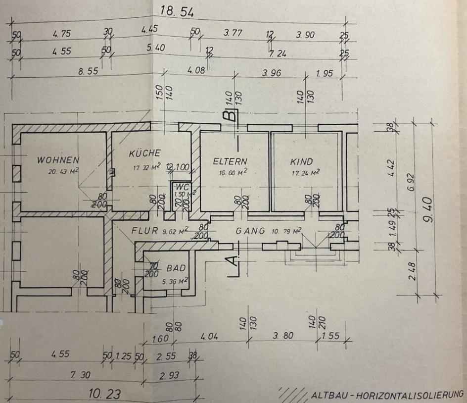
GRUNDRISS
