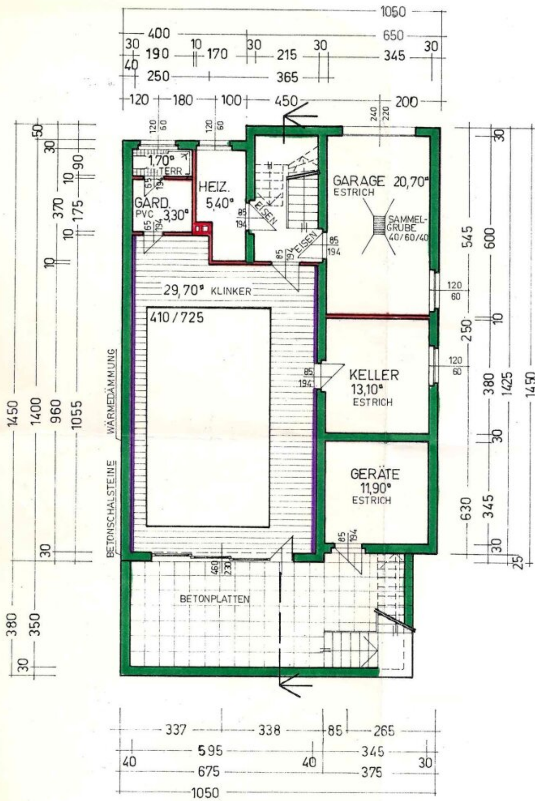
UNTERGESCHOSS
