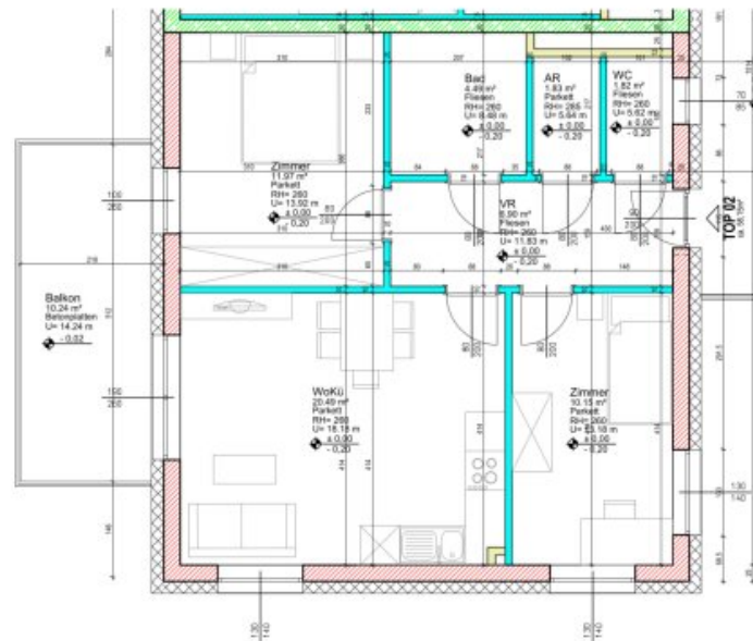
Planausschnitt 1.OBERGESCHOSS - Wohnung Planstand = Ausführungsplan M: 1:100
