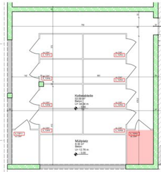
Planausschnitt KELLERGESCHOSS - Abteil TOP 02 - OST Planstand = Ausführungsplan M: 1:100
