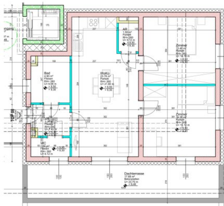
Planausschnitt 4.OBERGESCHOSS - Wohnung Planstand = Ausführungsplan M: 1:100
